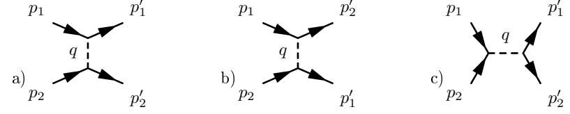
Рис. 1. Фейнманівські діаграми для процесів пружного розсіяння систем двох частинок.
