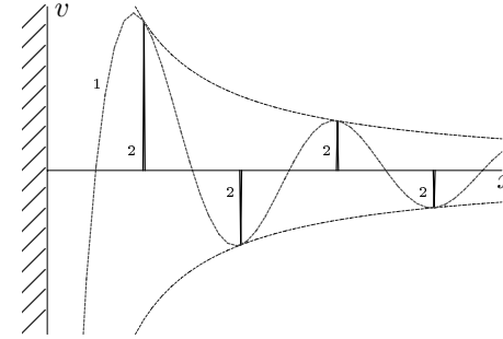
Рис. 6. 1. Тахіонний потенціал. 2. Еквівалентний діраківський гребінець.
