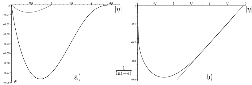
Рис. 5. Те ж, що на рис. 4, але для випадку “відштовхування” \alpha > 0 .
