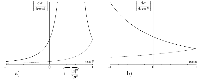
Рис. 2. Диференціальний перетин реакції 1+2 при масивному (пунктир) і тахійонному (суцільна крива) посередниках взаємодії з тим же значенням (мета)маси |\mu| : а) 2|\mathbf{p}| > |\mu| ; б) 2|\mathbf{p}| < |\mu| .
