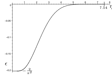
Рис. 7. Залежність енергії основного стану \epsilon від “метамаси” \eta модельного потенціалу (5.3)-(5.4). Зазначено мінімальну енергію та граничне значення метамаси.
