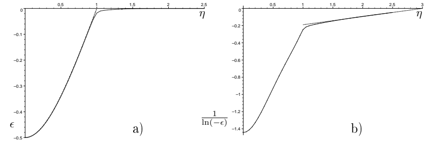
Рис. 4. а) залежність енергії основного стану від метамаси тахіонного посередника взаємодії (у безрозмірних змінних \epsilon , \eta ) для випадку “притягання” \alpha < 0 : суцільна крива – чисельні результати, пунктир – варіаційне наближення; б) асимптотична поведінка енергії при 1 < \eta < 3 .
