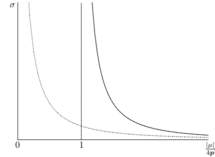
Рис. 2. Диференціальний перетин реакції 1+2 при масивному (пунктир) і тахійонному (суцільна крива) посередниках взаємодії з тим же значенням (мета)маси |\mu| : а) 2|\mathbf{p}| > |\mu| ; б) 2|\mathbf{p}| < |\mu| .
